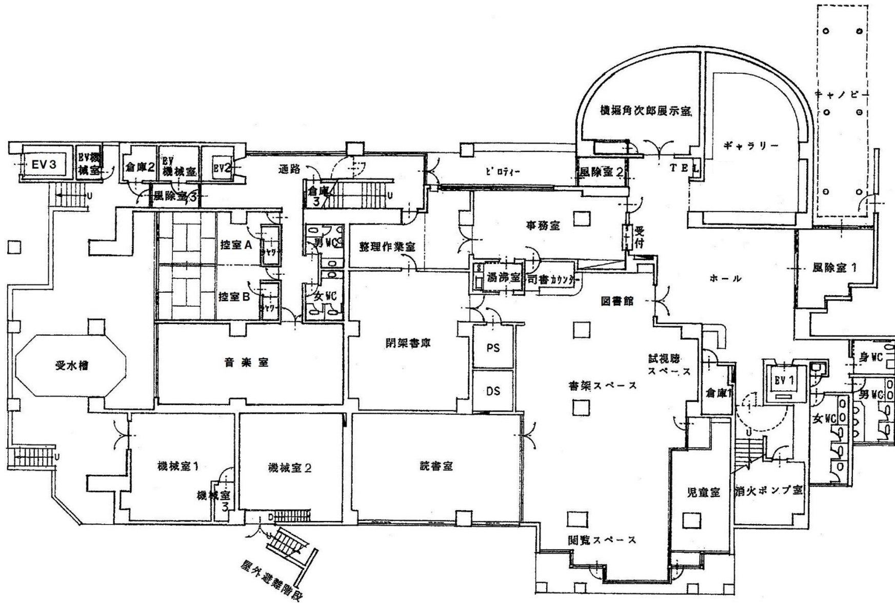
1階 平面図
